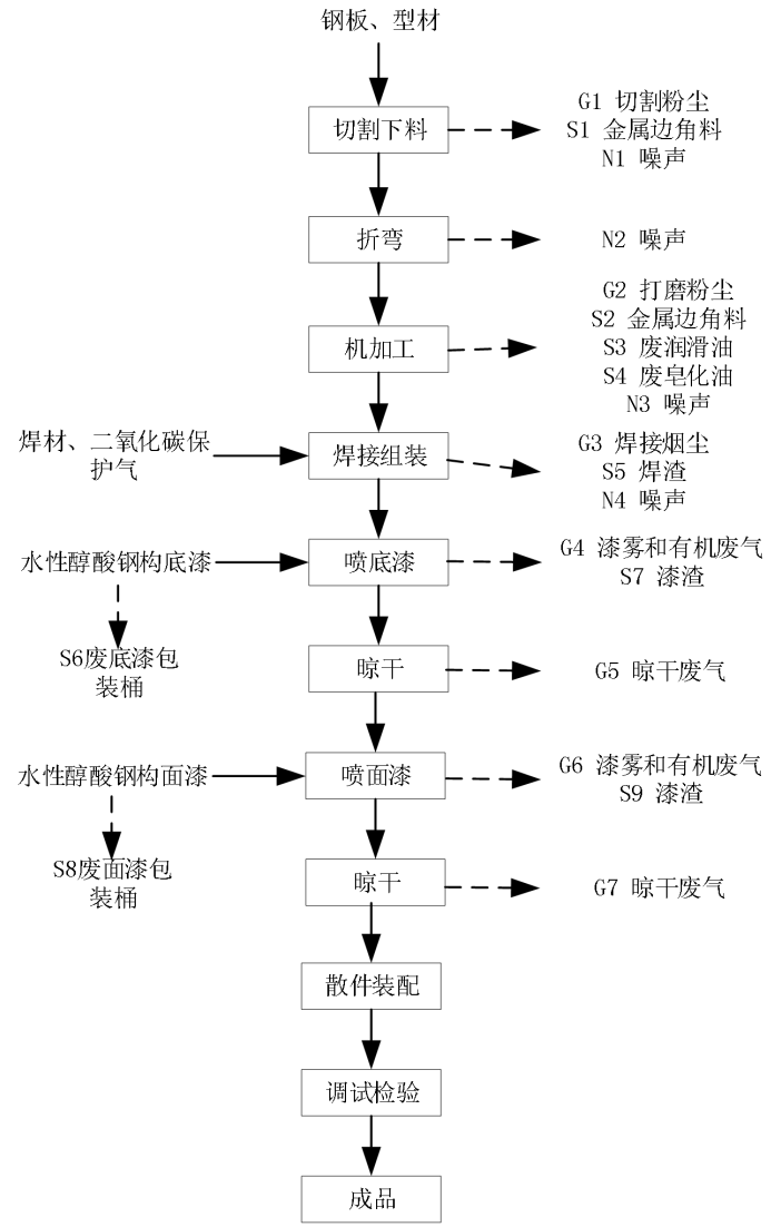
图 2-2 本项目生产工艺流程总图
